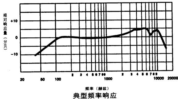
图 2 典型频率响应
