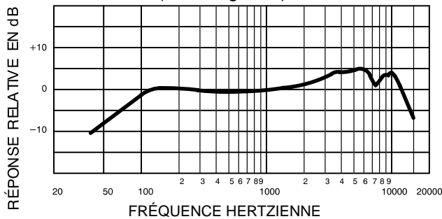
FRÉQUENCE HERTZIENNE COURBE DE RÉPONSE TYPIQUE FIGURE 2
